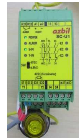
抵抗内蔵式(6.8kΩ)GS-M01接続 リセット前LED表示
