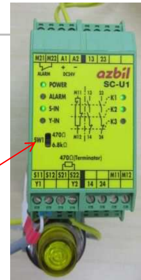
抵抗内蔵式(6.8kΩ)GS-M01接続 正常時(リセット後)LED表示
